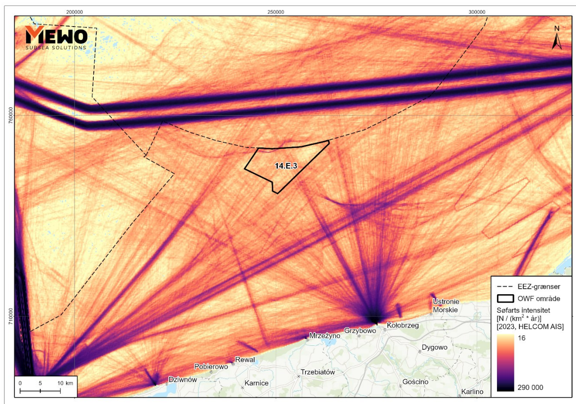
Figur 2.3 Placering af OWF 14.E.3 i forhold til alle fartøjers udnyttelse af havområdet. AIS-data – gennemsnit for 2023 (kilde: egen undersøgelse baseret på EMODnet-data)
