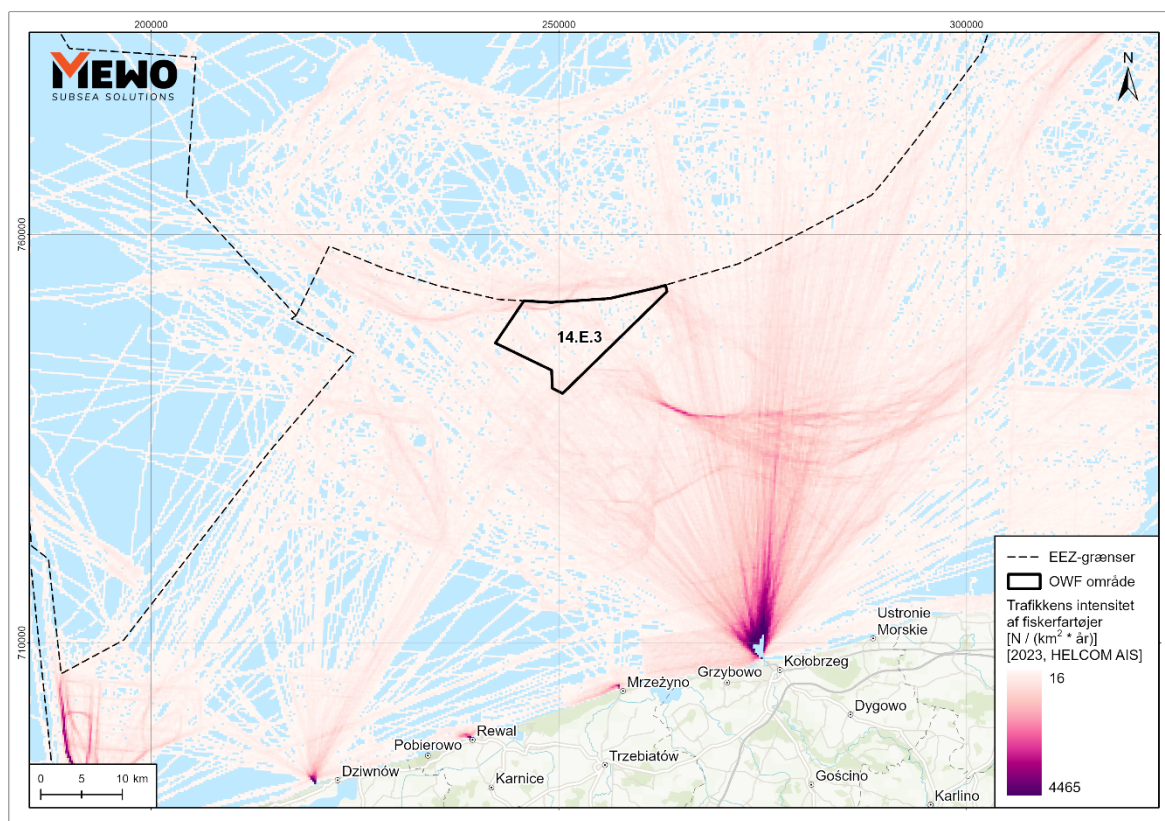
Figur 2.4 Placering af OWF 14.E.3 i forhold til fiskerfartøjers brug af havområdet. AIS-data – gennemsnit for 2023 (kilde: egen undersøgelse baseret på EMODnet-data)
