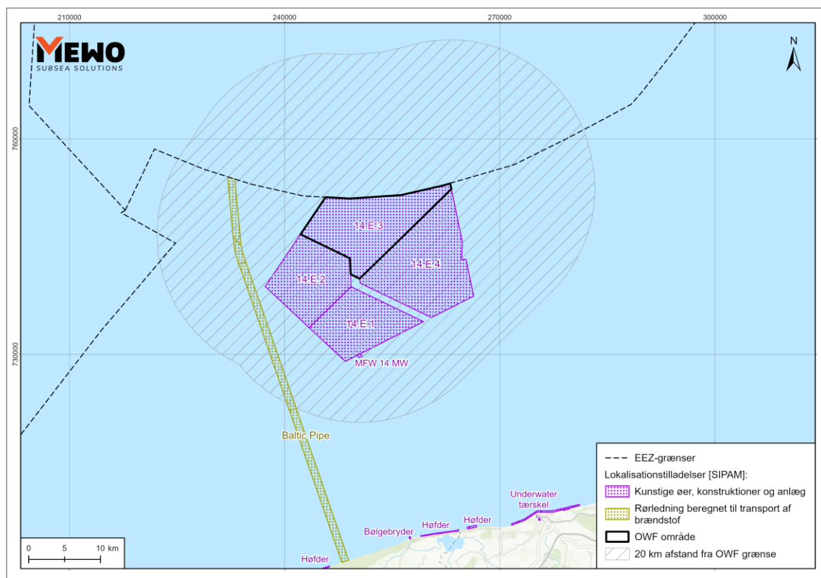
Figur 10.1. Placering af projekter planlagt til implementering uden for OWF 14.E.3 område, som kan være inden for projektets påvirkningsområde, eller hvis påvirkninger kan kumuleres med påvirkningerne fra OWF 14.E.3. (kilde: egen undersøgelse baseret på
