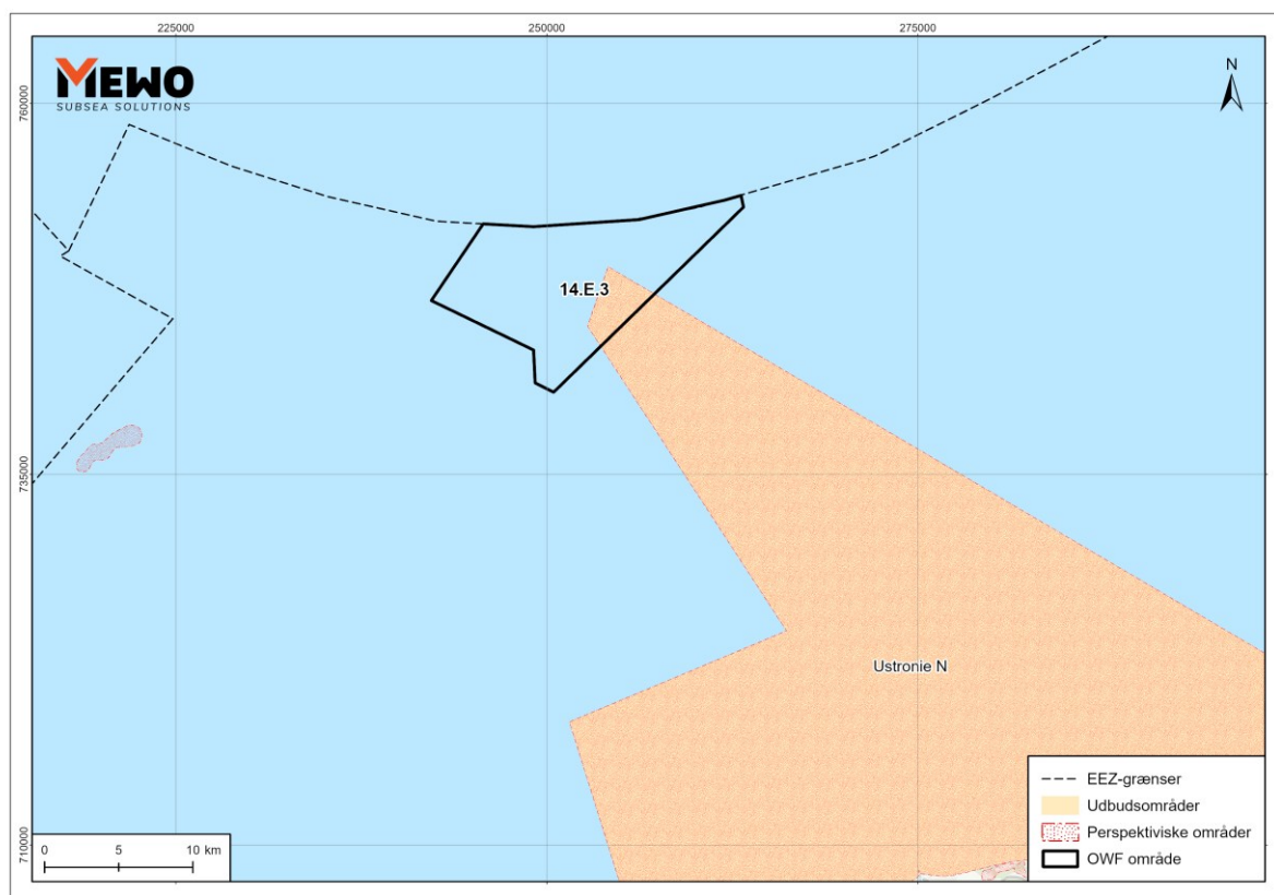
Figur 2.6 . Placering af OWF 14.E.3 i forhold til udbuds- og "perspektiv områder" (kilde: egen undersøgelse baseret på information fra den centrale geologiske database)
